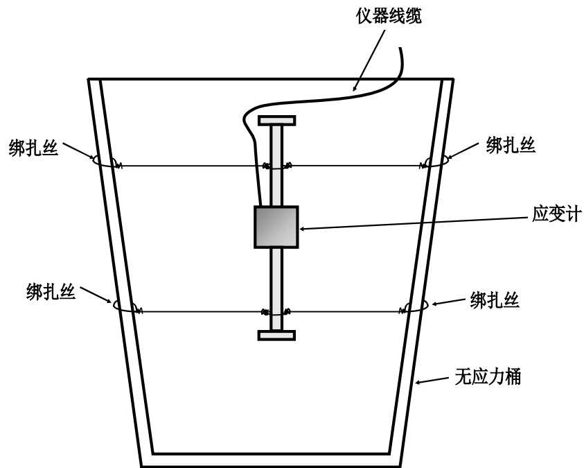
图 5 - 无应力桶预制块安装
