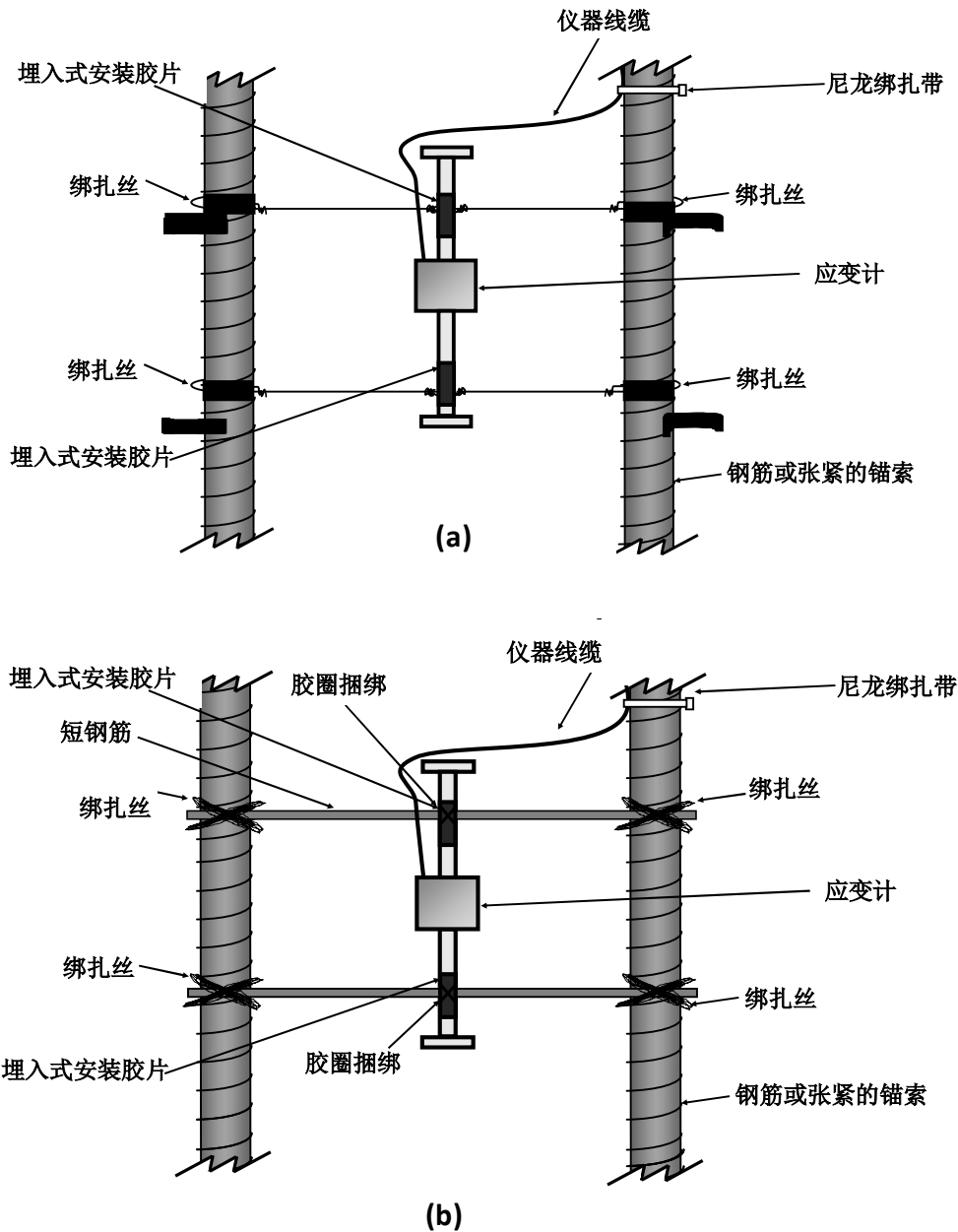
图 4 - 两根钢筋间安装示意图
