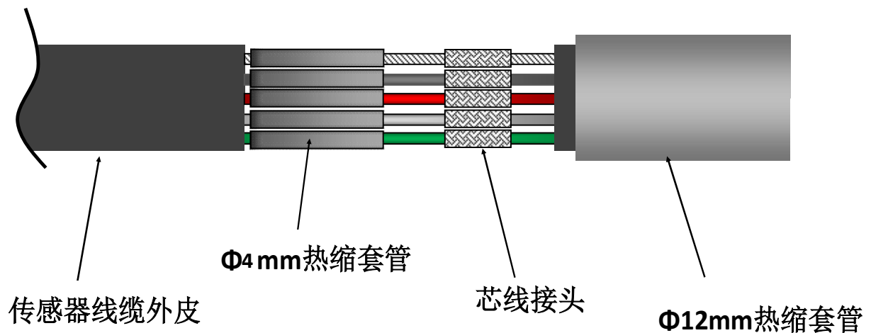
图 2 - 线缆焊接示意图
