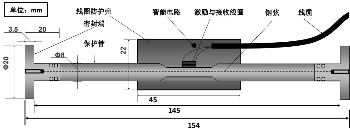
图 1 - TVA01A 产品结构示意图
