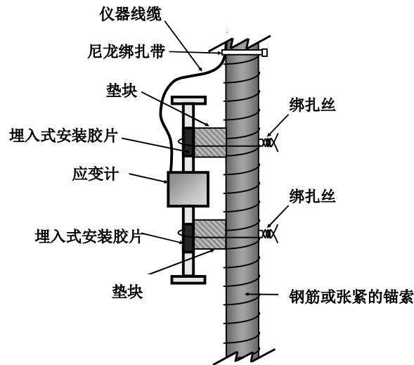
图 3 - 单根钢筋、锚索安装
